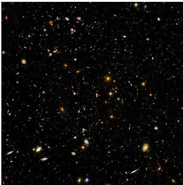
Рис. 2 Hubble Ultra-Deep Field – фотографии Вселенной, охватывающие области сверхглубокого космоса, сделанные космическим телескопом “Хаббл”.
