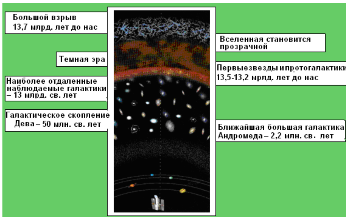
Рис.3 Большой взрыв по последним данным должен был совершиться 13,7 млрд. лет тому назад. Космический телескоп “Хаббл” позволяет нам достичь почти “границы” Вселенной.
